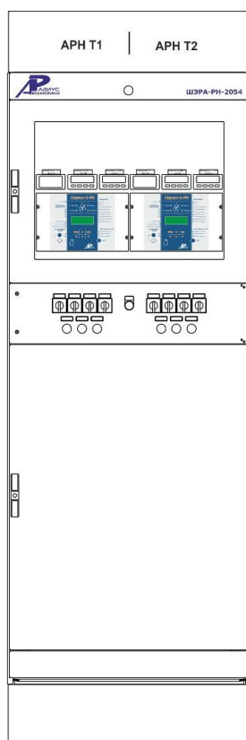
Шкаф регулирования напряжения двух трансформаторов (АТ) ШЭРА-РН-2054 БПВА.656457.165, БПВА.650645.001 ТУ
